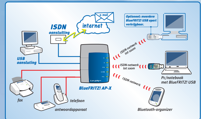
BlueFRITZ! AP-X
