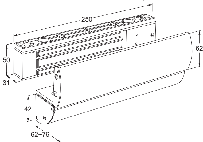
17ZLC Z en L steun met afdekkap voor een naar binnen draaiende deur
