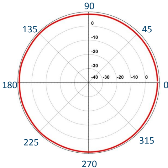
H-Plane
